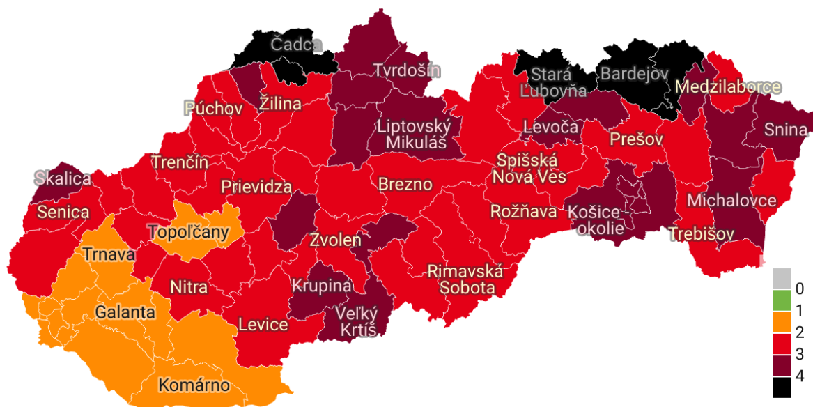
Obrázok 1 - Covid Automat pre 42KT (18.10. – 24.10.2021)
